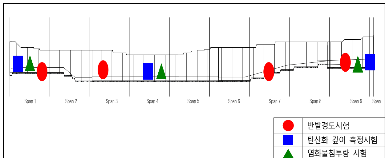
【그림 81.6】 콘크리트 재료시험 조사 위치도
