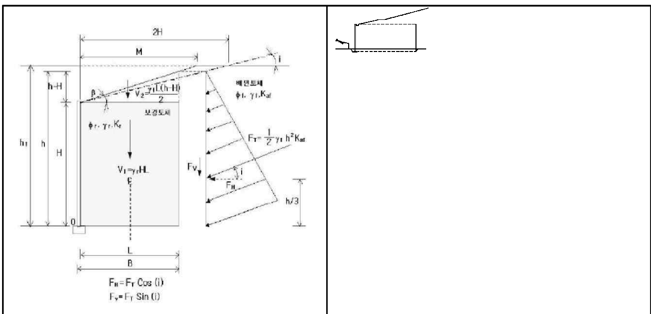
【그림 81.11】 토압작용 모식도
