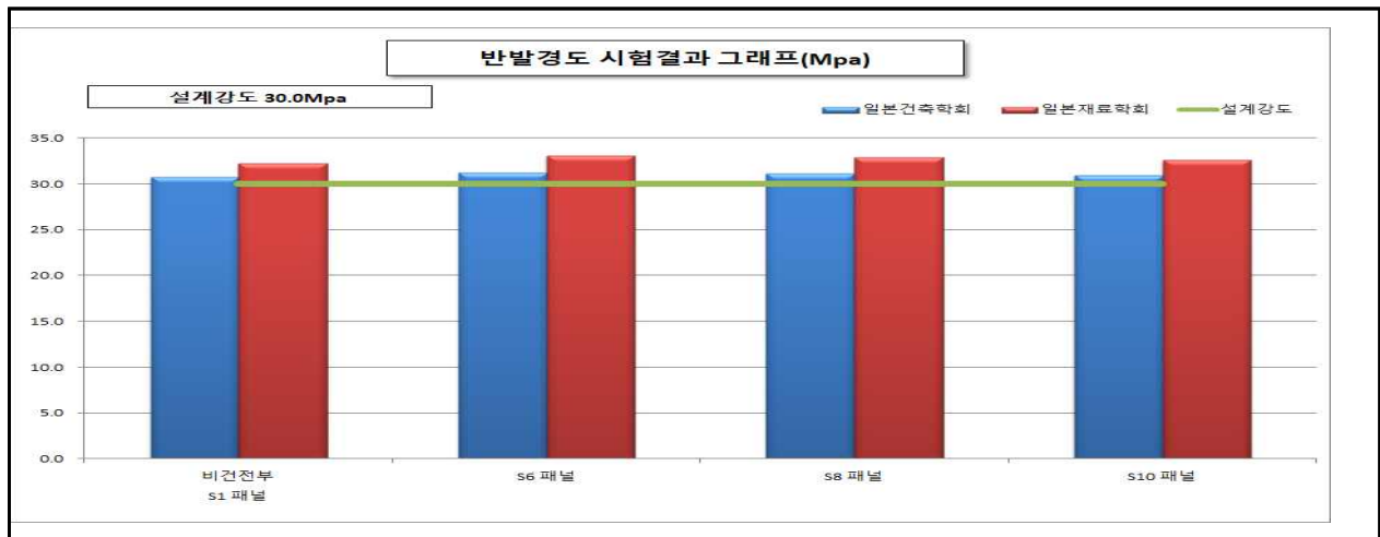
【그림 81.7】 반발경도시험 측정결과
