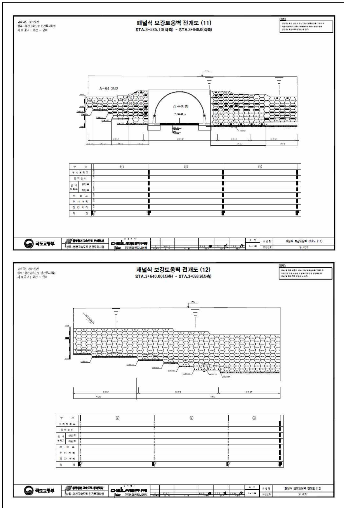
【그림 81.4】 전개도
