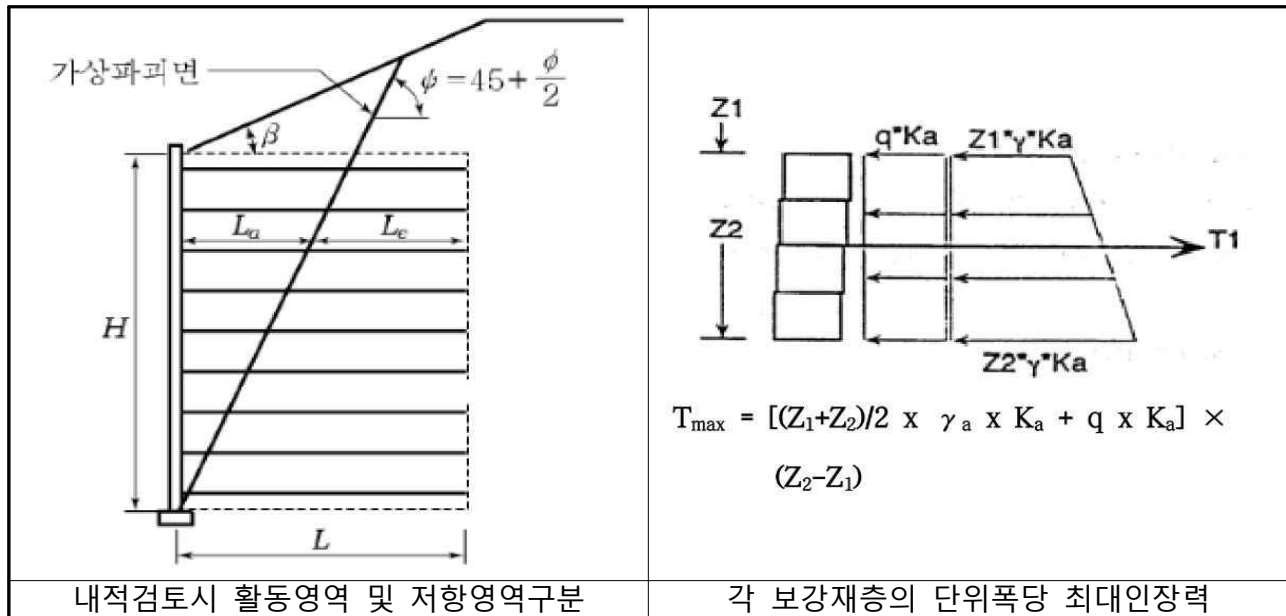
【그림 81.12】 토압작용 모식도
